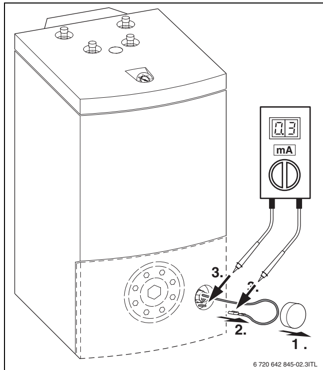
Рис. 7 Проверка анода
