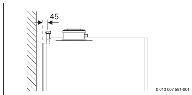
Рис. 8 Присоединительные размеры дополнительного оборудования CS11 комплект для вертикального подключения (в мм)
