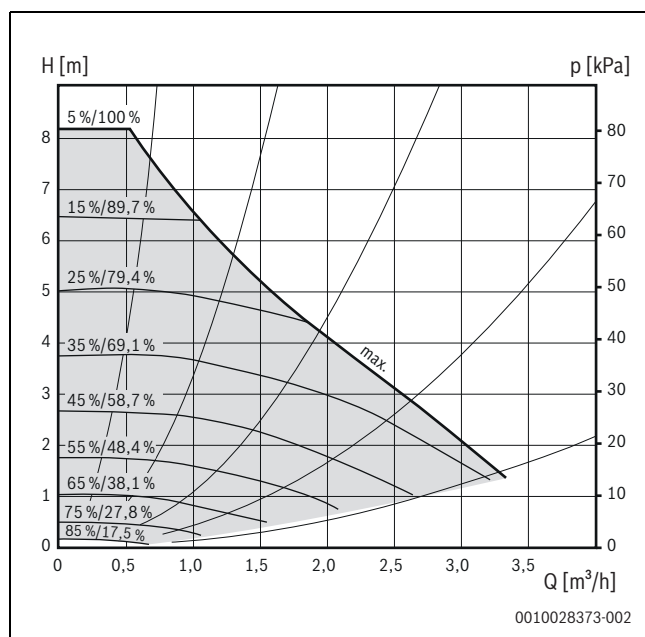
Рис. 122 Поля характеристик и характеристические кривые насоса солнечной установки Para ST 15/7-50/iPWM 2, диапазон частоты вращения 20–100 %, диапазон производительности 0–16,5 л/мин
