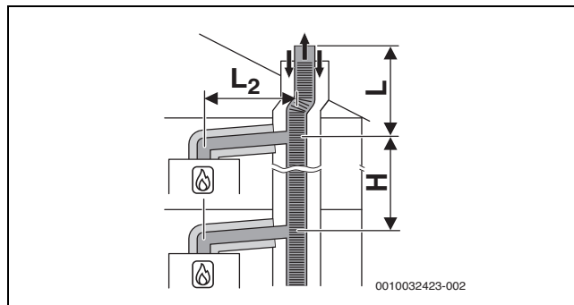
Рис. 40 Подключение нескольких котлов к одной дымовой трубе по C_{(14)3x} с коллективным гибким отводом дымовых газов и концентрическим подводом воздуха/отводом дымовых газов в помещении установки оборудования
