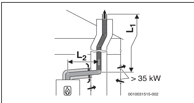
Рис. 37 Схема гибкого отвода дымовых газов в шахте согласно V 33 с забором воздуха из помещения через концентрический подвод воздуха/отвод дымовых газов в помещении для установки
