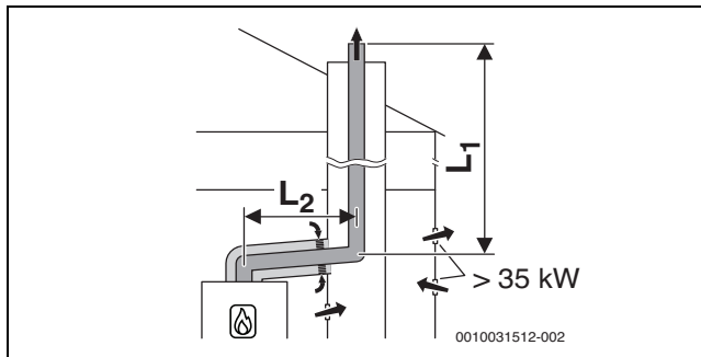
Рис. 36 Схема жесткого отвода дымовых газов в шахте согласно V 33 с забором воздуха из помещения через концентрический подвод воздуха/отвод дымовых газов в помещении для установки
