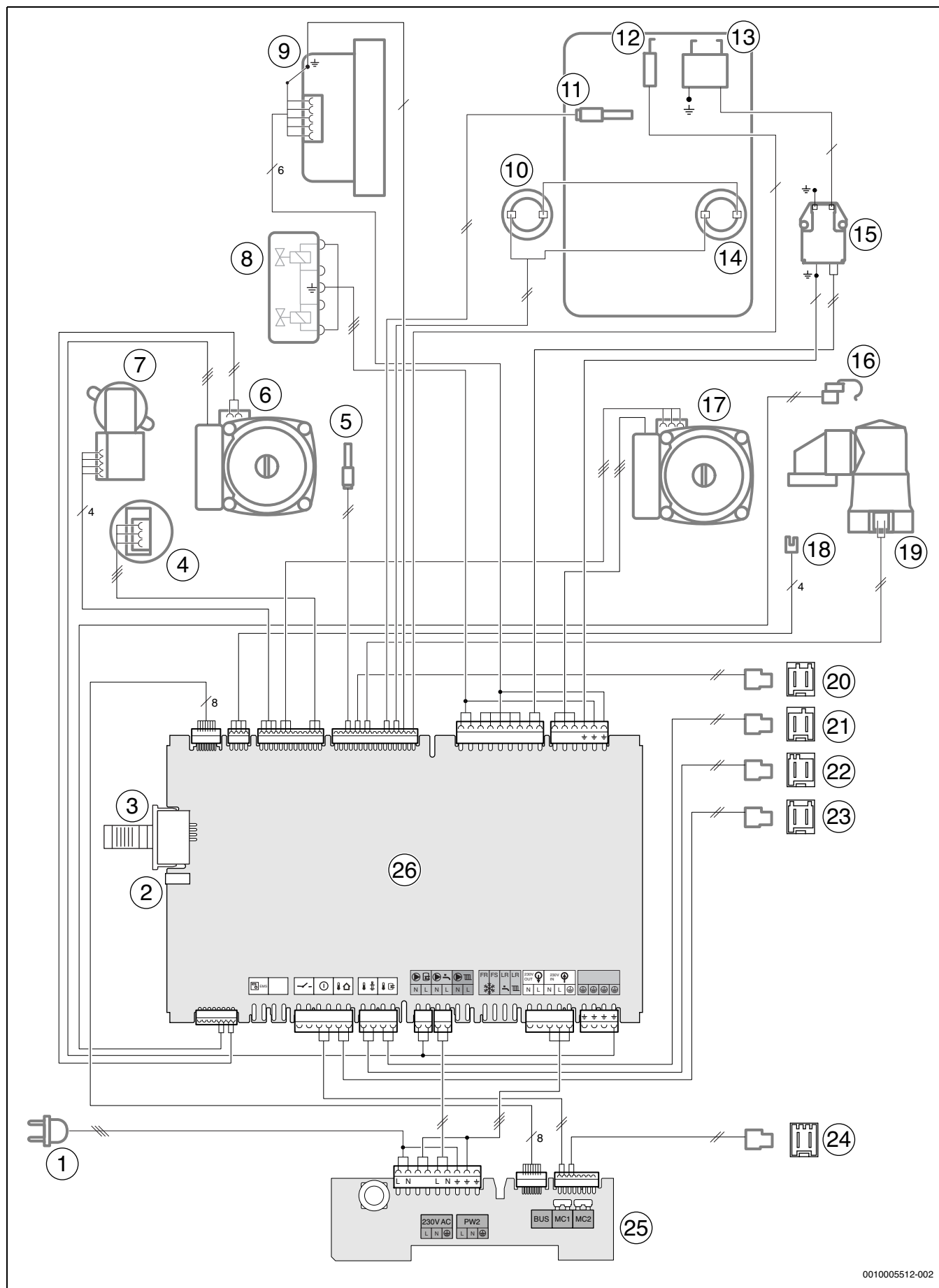
Рис. 120 Электрические соединения
