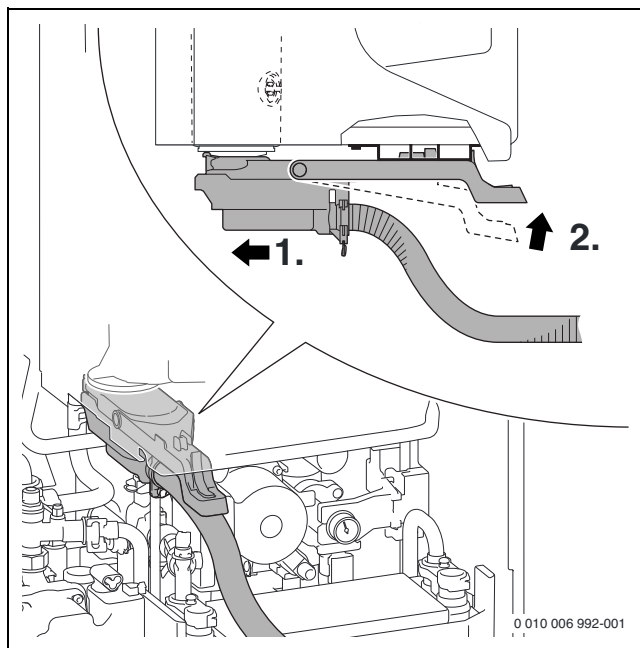
Рис. 56 Смонтируйте грязеуловитель
