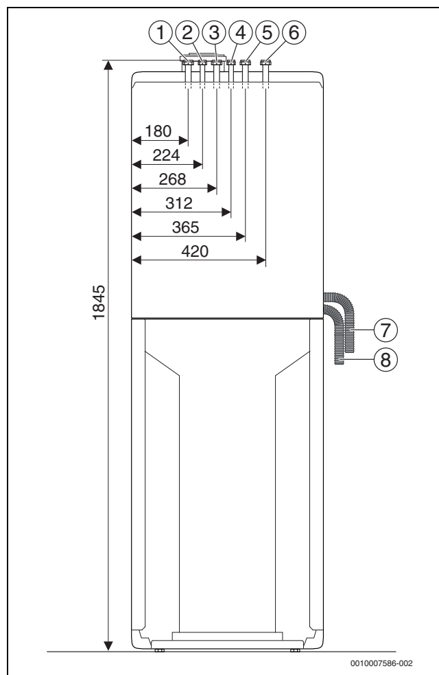
Рис. 7 Присоединительные размеры дополнительного оборудования CS11 комплект для вертикального подключения (в мм)
