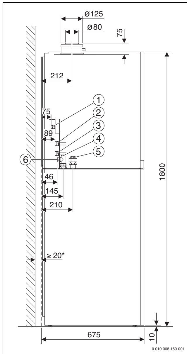
Рис. 2 Размеры и подключения без дополнительного оборудования (в мм)
