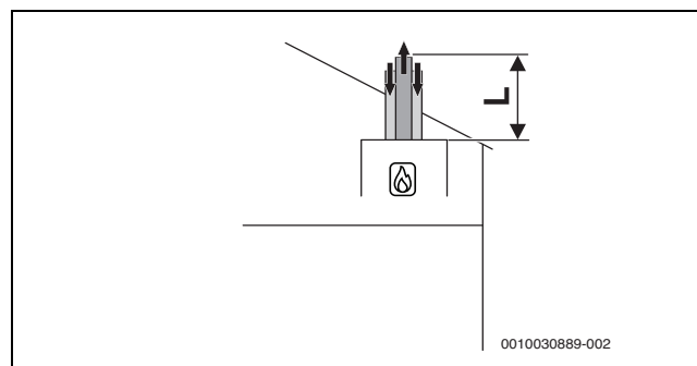
Рис. 26 Вертикальная концентрическая схема подачи воздуха/отвода дымовых газов согласно C_{33x}
