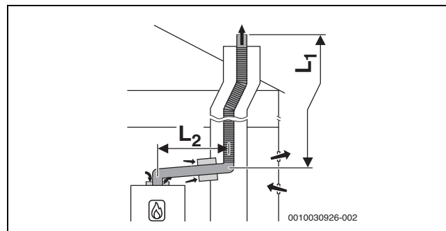
Рис. 35 Схема гибкого отвода дымовых газов в шахте согласно B 23p /B 53p с забором воздуха из помещения топочной для подвода воздуха и с концентрическим соединительным элементом между помещением для установки и шахтой
