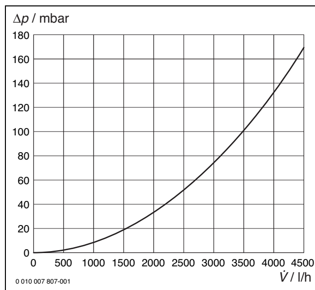
Рис. 124 Диаграмма потерь давления отопительного контура со смесителем (HK2)
