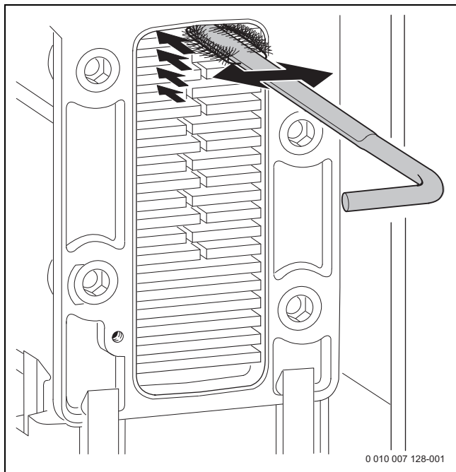
Рис. 104 Очистка теплообменника щёткой
