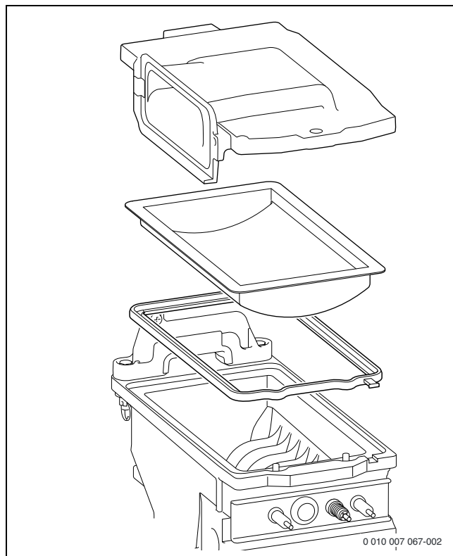
Рис. 102 Горелка
