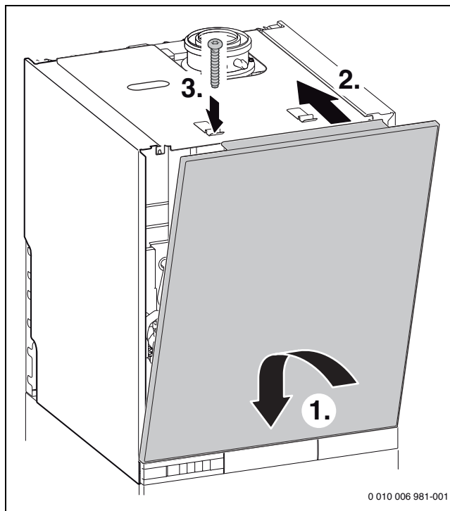
Рис. 87 Установка передней облицовки и крепление винтом из комплекта поставки
