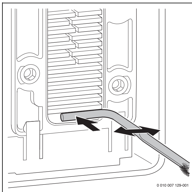
Рис. 106 Очистка конденсатной ванны
