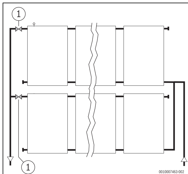
Рис. 81 Промывка параллельно подключенных полей коллекторов
