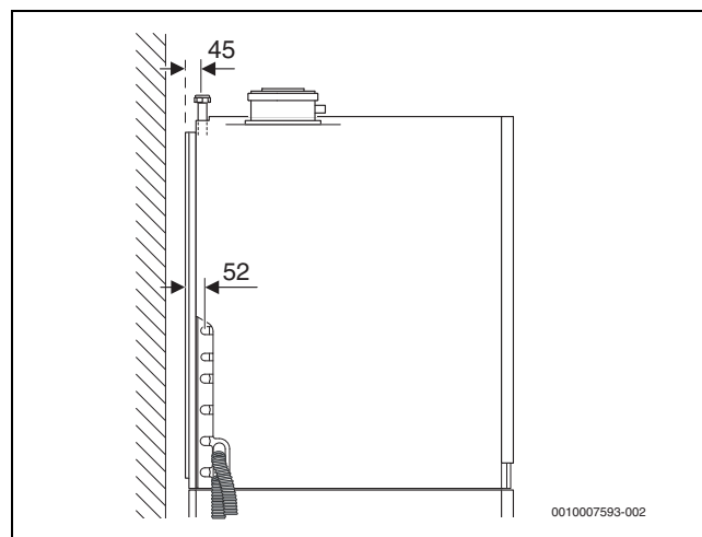
Рис. 10 Присоединительные размеры дополнительного оборудования CS12 расширение отопительного контура 1 (в мм)
