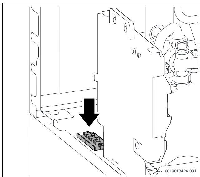
Рис. 63 Закрепите на баке колодку штекерных разъемов
