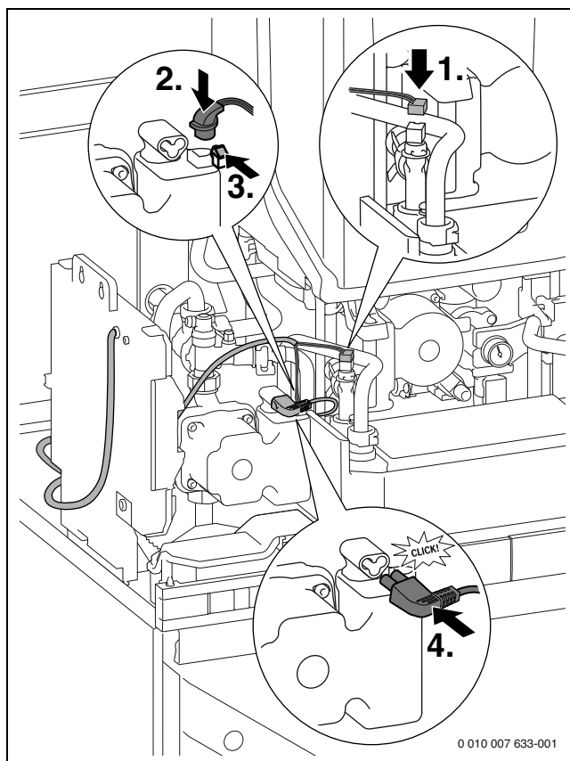
Рис. 64 Подключите датчик температуры горячей воды и загрузочный насос бака
