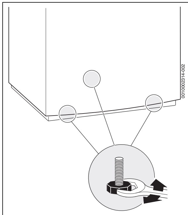
Рис. 52 Выравнивание бака
