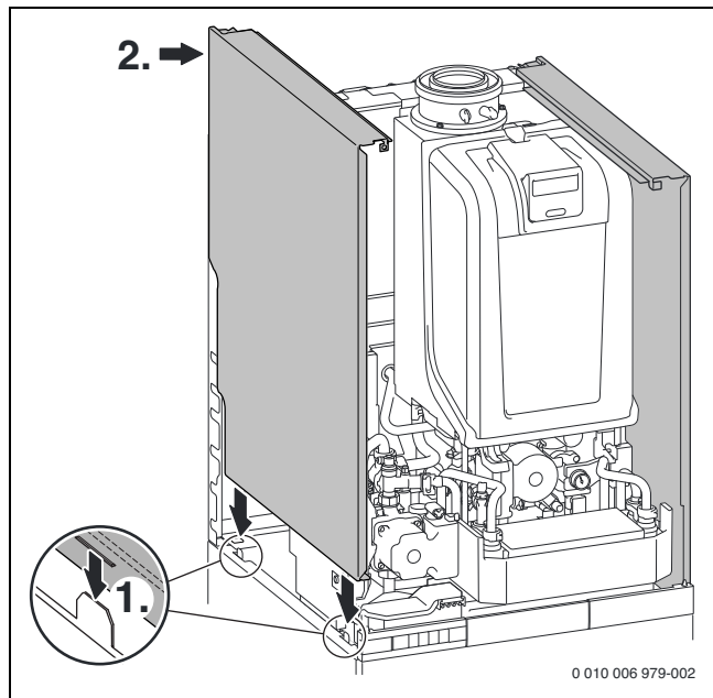
Рис. 85 Монтаж правой и левой облицовки
