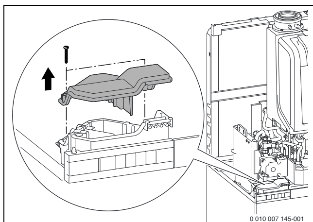
Рис. 66 Снимите крышку клеммной коробки
