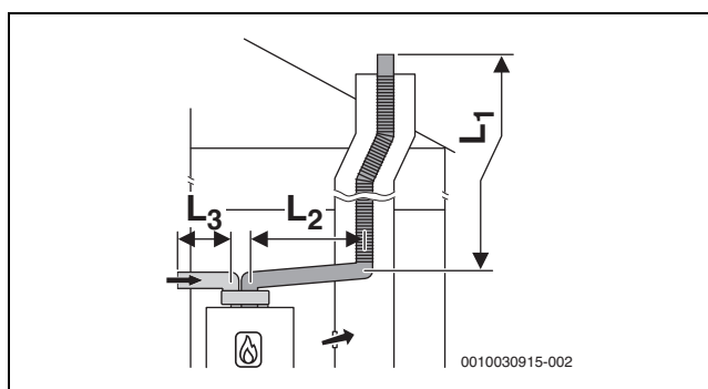
Рис. 30 Схема гибкого отвода дымовых газов согласно C 53 в шахте и схема подачи воздуха/отвода дымовых газов отдельными трубами для линии подвода воздуха и линии отвода дымовых газов в помещении для установки
