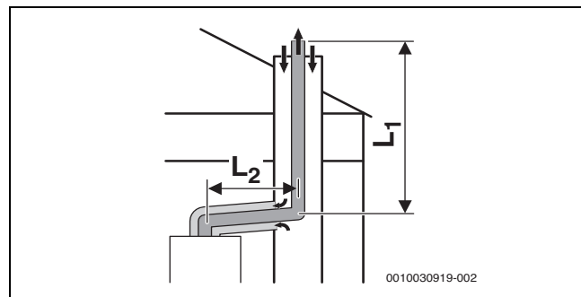
Рис. 32 Схема жесткого отвода дымовых газов согласно C_{93x} в шахте и концентрический подвод воздуха/отвод дымовых газов в помещении для установки
