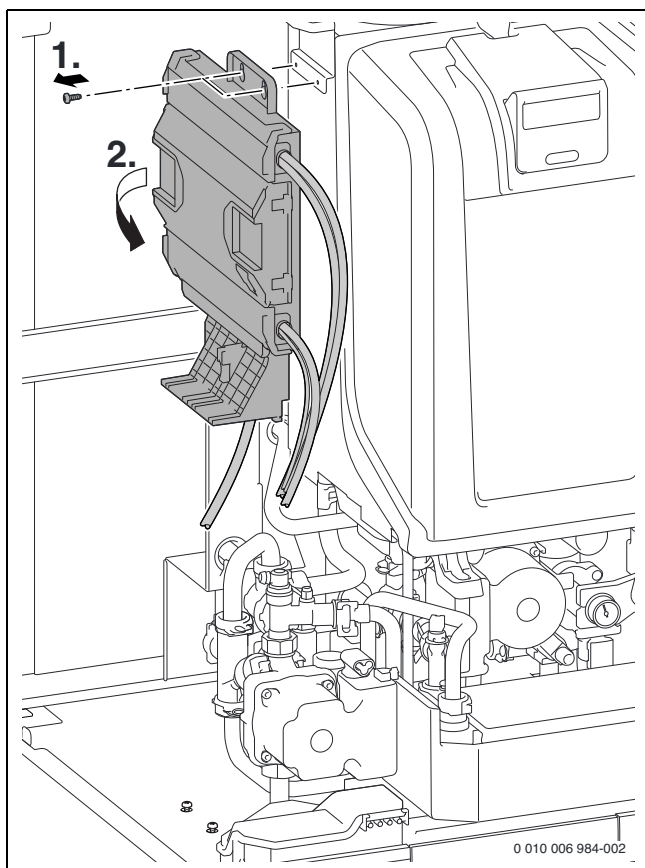
Рис. 61 Снимите блок управления
