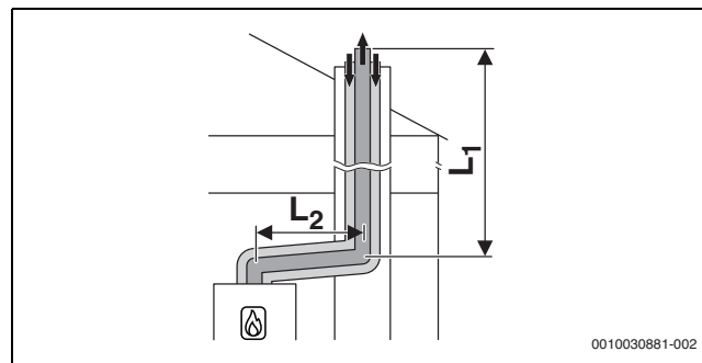
Рис. 25 Концентрическая схема подачи воздуха/отвода дымовых газов согласно C_{33x} в шахте
