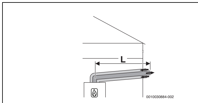
Рис. 22 Горизонтальная концентрическая схема подачи воздуха/отвода дымовых газов согласно C_{13x} через наружную стену
