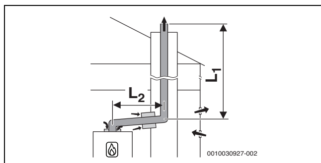
Рис. 34 Жёсткий отвод дымовых газов в шахте по B 23p /B 53p с забором воздуха из помещения и с концентрическим соединительным элементом между помещением установки котла и шахтой
